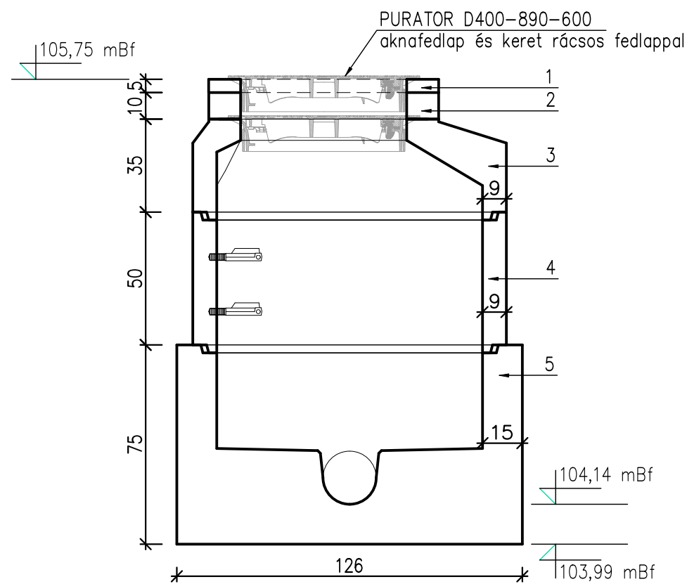
Sz-1 szennyvíz csatorna 2 jelű akna 0+036,5
