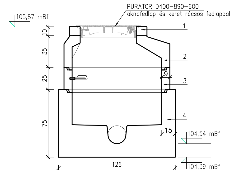
Sz-1 szennyvíz csatorna 5 jelű akna 0+116,5
