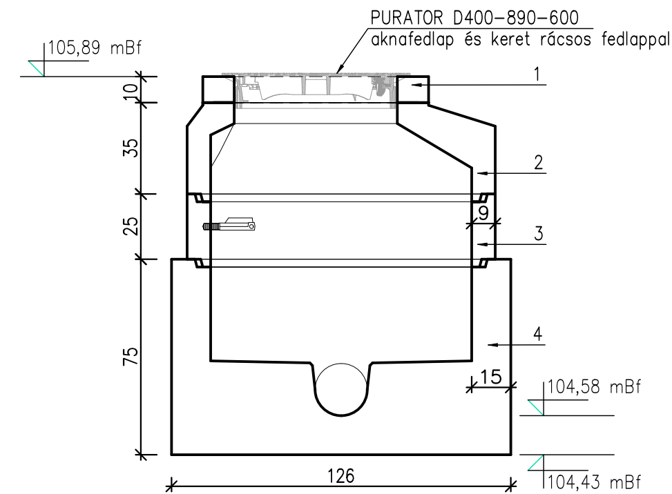
Sz-1 szennyvíz csatorna 6 jelű akna 0+123,0
