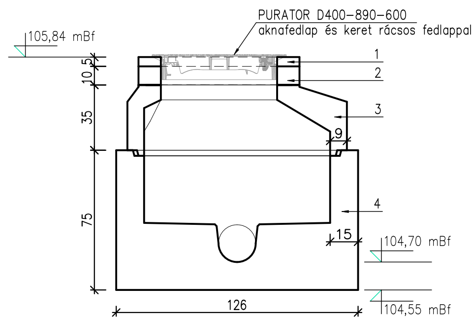
Sz-1 szennyvíz csatorna 7 jelű akna 0+148,5
