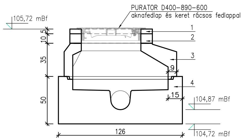
Sz-1 szennyvíz csatorna 9 jelű akna 0+033,4
