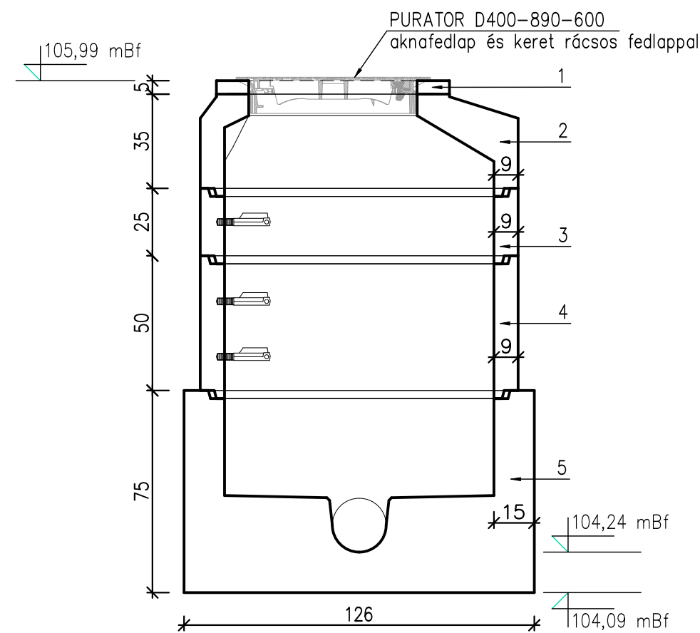
Sz-1 szennyvíz csatorna 3 jelű akna 0+056,5
