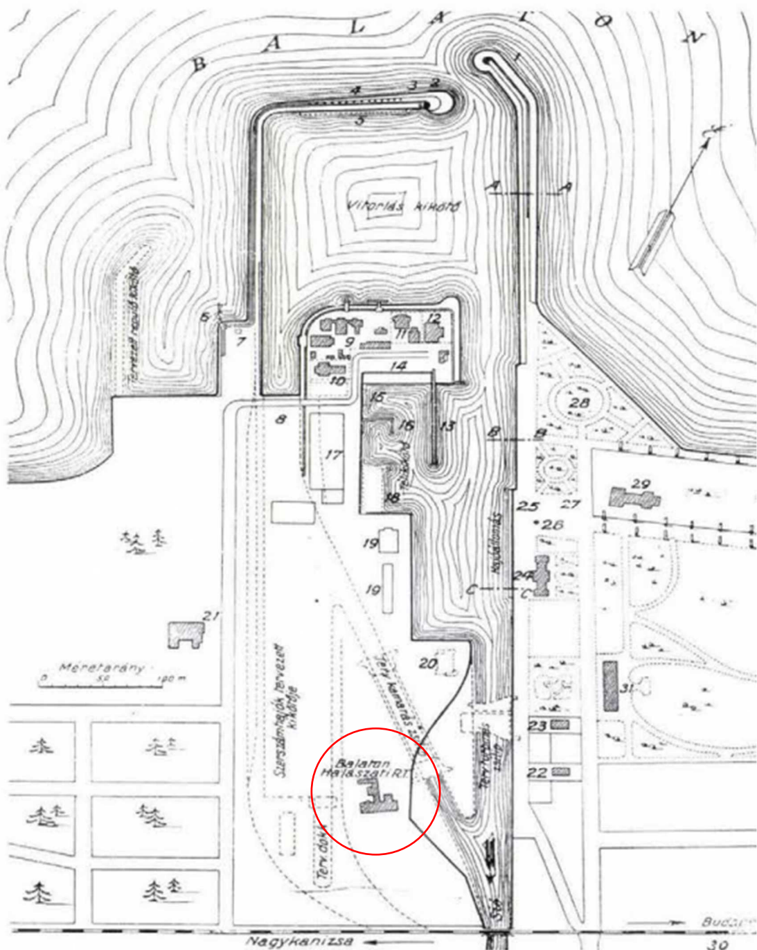
A siófoki kikötő és a Sió torkolati-mű Kaáli Nagy Dezső-féle terve (a Lampl Hugó és Pataky Béla által közöltek szerint)
